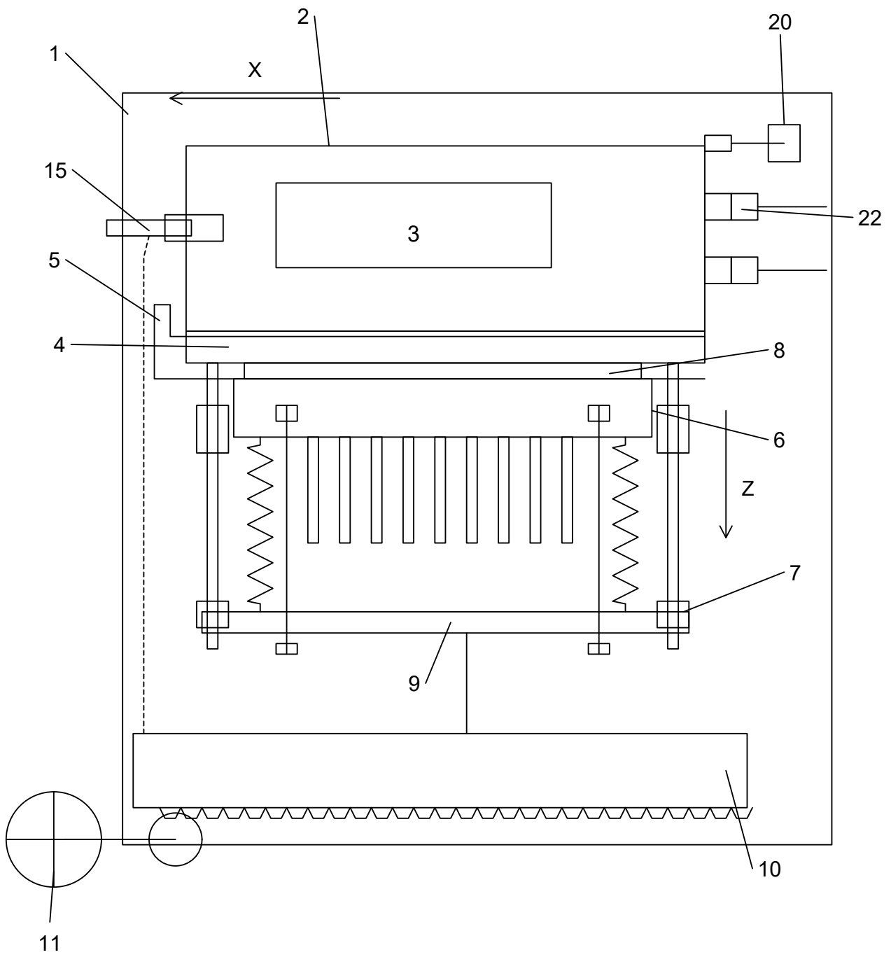
Продольный разрез. Сервисный привод — в проекции.
